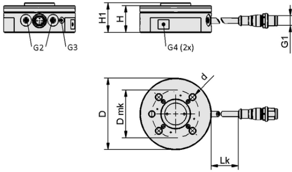
Tasarım verileri RMQC 50 FANUC DIO WB-M8-8 PNP MATCH
