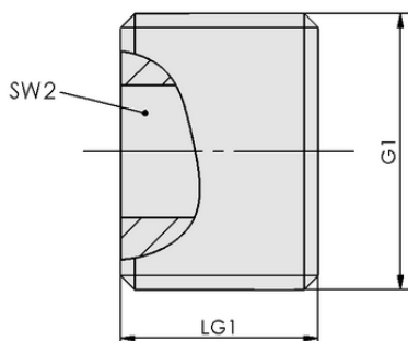
デザインデータ VRS-S G3/8-AG
