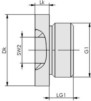
Tasarım verileri VRS-SB G1/4-AG ISKT O-Ring
