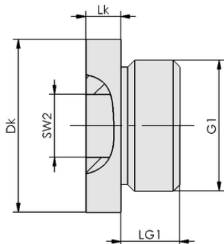
Design data VRS-SB G1/4-AG ISKT O-Ring
