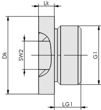
Tasarım verileri VRS-SB G1/8-AG ISKT O-Ring
