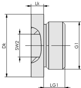
デザインデータ VRS-SB M5-AG SKT
