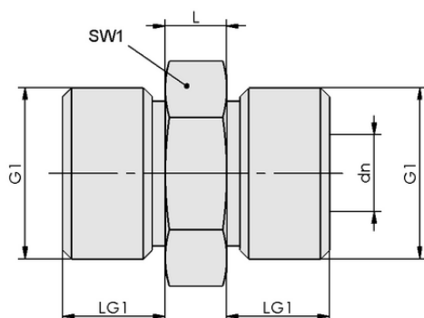
Données de construction DOP-NIP-S G1/2-AGx6
