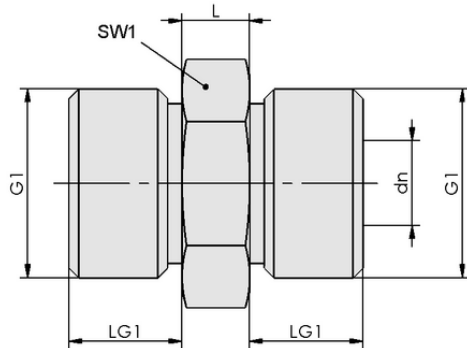
デザインデータ DOP-NIP-S G3/8-AGx5
