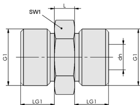
デザインデータ DOP-NIP-S G1/4-AGx5
