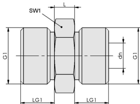
デザインデータ DOP-NIP-S G1/8-AGx5
