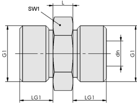
Tasarım verileri DOP-NIP-S M5-AGx4
