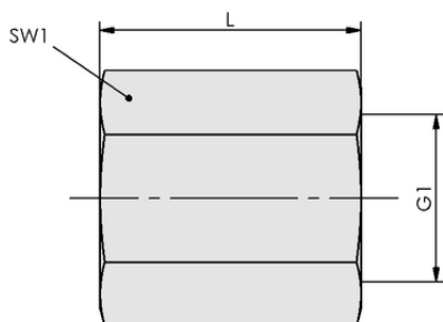
デザインデータ MUF-S G1-IG 33 SW41 MS-VN
