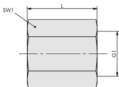
デザインデータ MUF-S G1/8-IG 18 SW14 MS-V
