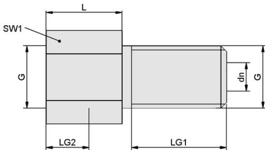
デザインデータ VRL-S G1/2x22 MS-V
