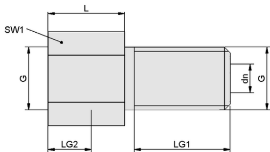
デザインデータ VRL-S M5x8 MS-V
