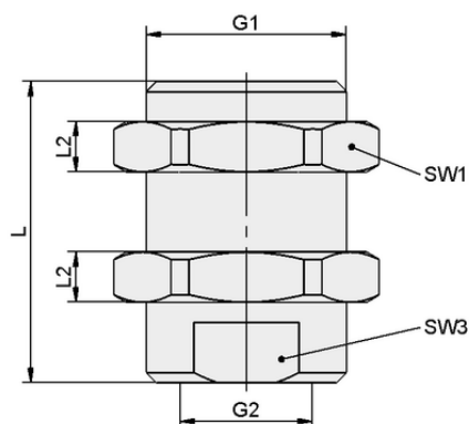
Datos de diseño SVS-GE M30x1.5-AG G1/2-IG 40
