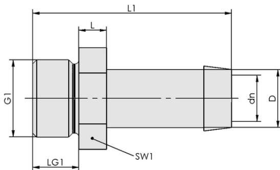
Konstruktionsdaten ST M5-AG 2.5 MS-V
