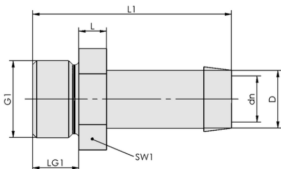
Données de construction ST M5-AG 2.5 MS-V
