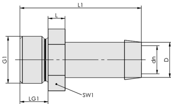
Konstruktionsdaten ST M5-AG 4 MS-V
