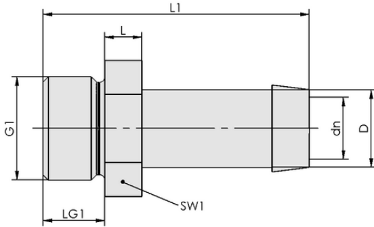
Tasarım verileri ST G3/4-AG 25 MS-V
