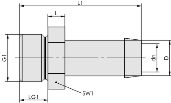
Tasarım verileri ST G3/4-AG 19 MS-V
