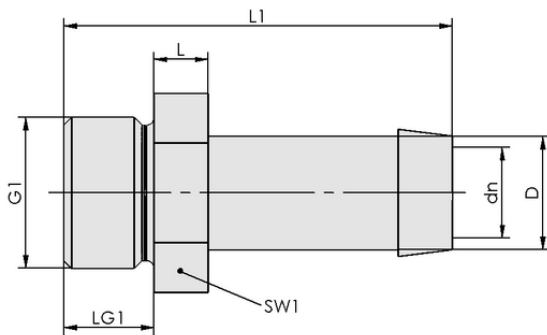
Datos de diseño ST G1/4-AG 13 MS-V
