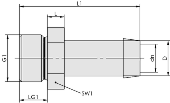
Tasarım verileri ST G1/4-AG 6 MS-V
