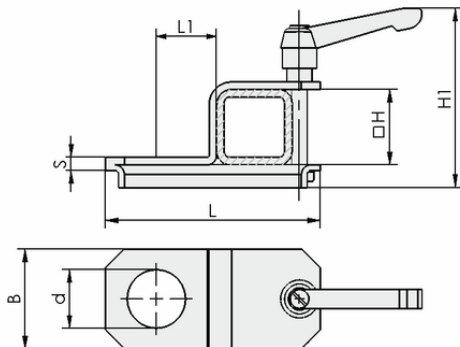
Konstruktionsdaten HTR-STS 50x50 D30 WI
