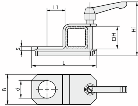
Tasarım verileri HTR-STS 50x50 D30 WI
