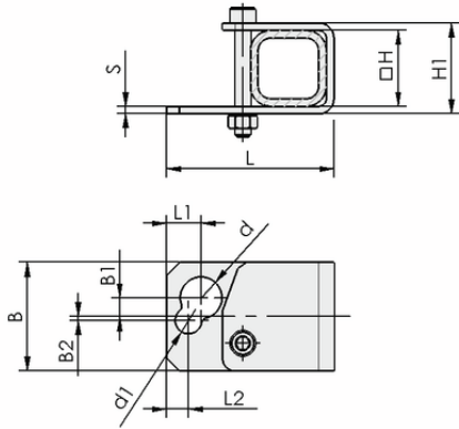
Tasarım verileri HTR-STS 40x40 D10/16 WI
