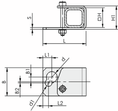
Tasarım verileri HTR-STS 30x30 D10/16 WI
