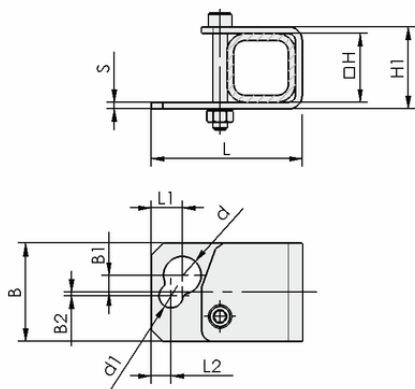
Design data HTR-ST5 30x30 D10/16 WI
