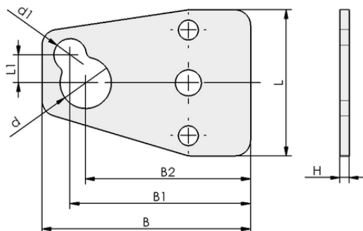
Design data HTR-STA 47 1N D10/16 FL
