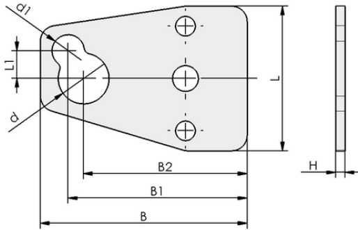
Tasarım verileri HTR-STA 47 1N D10/16 FL
