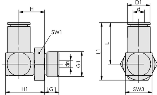
Tasarım verileri STV-W G1/2-AG 10
