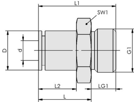
Tasarım verileri STV-GE G1/4-AG 10
