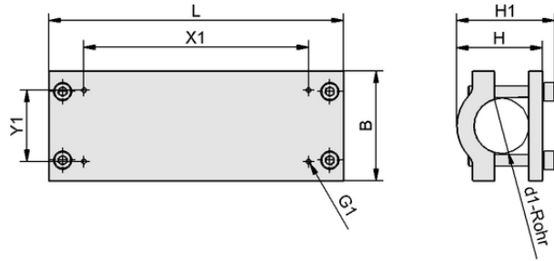
Tasarım verileri SXT-CL-MP D 40 215
