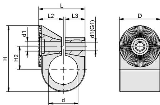
Données de construction SXT-CON-GB-M-A2
