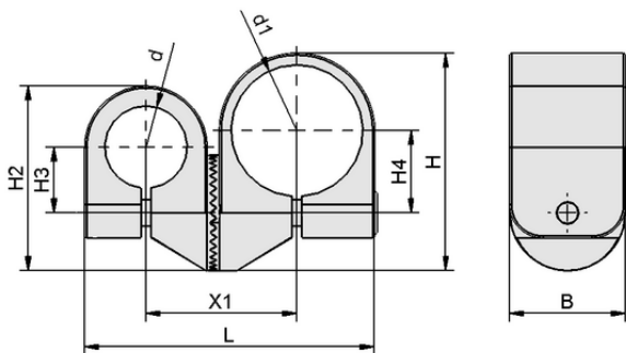
Datos de diseño SXT-TC-F2-0-C1.5IN
