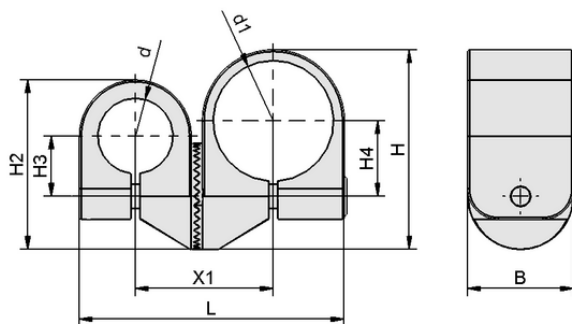
デザインデータ SXT-TC-F4-0-M4
