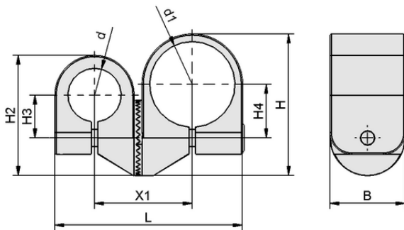
Données de construction SXT-TC-F2-0-M4
