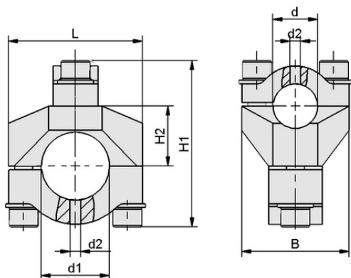
Dati di costruzione SXT-CL X MOD 25 AL 1IN
