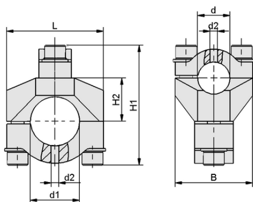
Données de construction SXT-CL X MOD 25 AL 1IN
