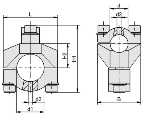
Datos de diseño SXT-CL X MOD 25 AL 1IN
