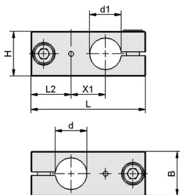
Dati di costruzione SXT-CL X FIX 40 60 AL
