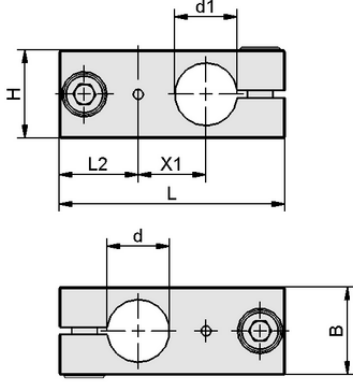
Tasarım verileri SXT-CL X FIX 40 60 AL
