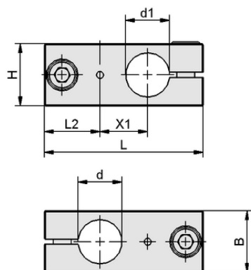
デザインデータ SXT-CL X FIX 40 60 AL
