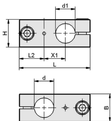
Datos de diseño SXT-CL X FIX 40 40 AL
