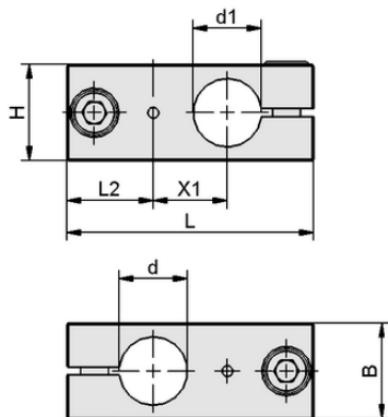
Datos de diseño SXT-CL X FIX 25 40 AL
