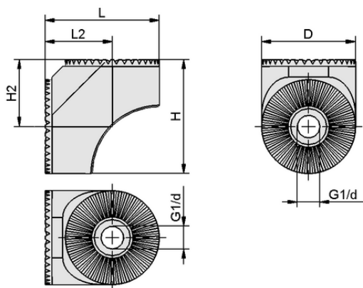
Datos de diseño SXT-ANG-GB2-F
