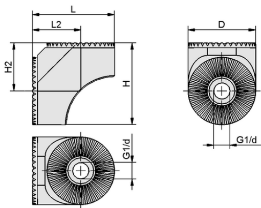
Données de construction SXT-ANG-GB2-M
