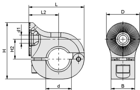
Données de construction SXT-CON-GB-MO-D40
