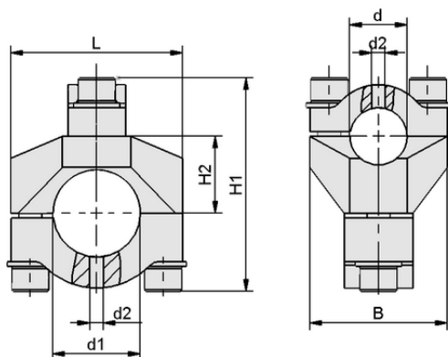
Données de construction SXT-CL X MOD 40 40 AL
