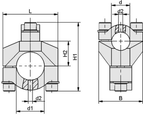
Tasarım verileri SXT-CL X MOD 25 40 AL
